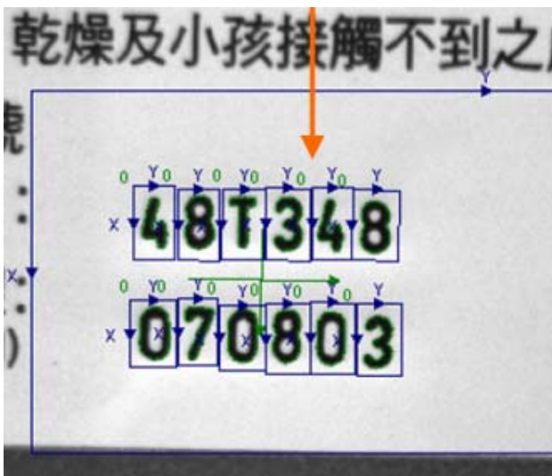
正常標籤影像參考線對準 3
